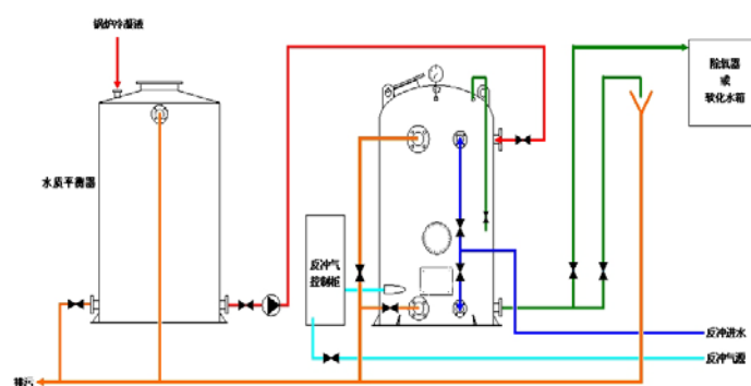
除铁过滤器流程图
