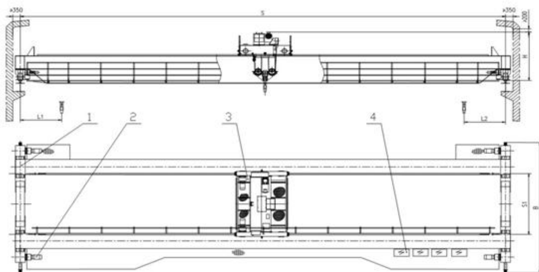
轻量化桥式起重机结构简图
