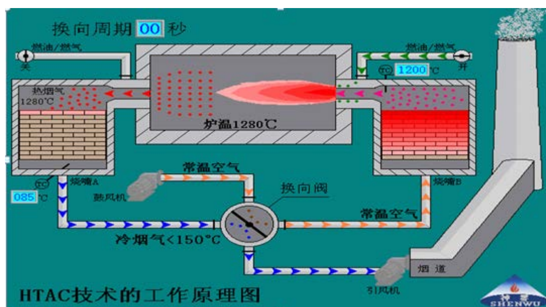
图 1 蓄热式燃烧器的工作原理图
