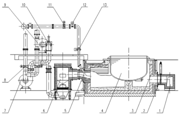
图 3-1 铅熔炼节能技术结构示意图
