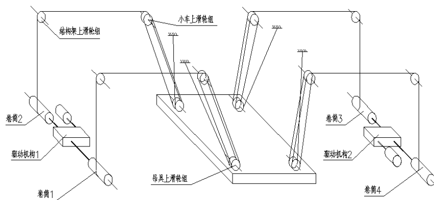
图1 “四卷筒”组合驱动原理示意图
