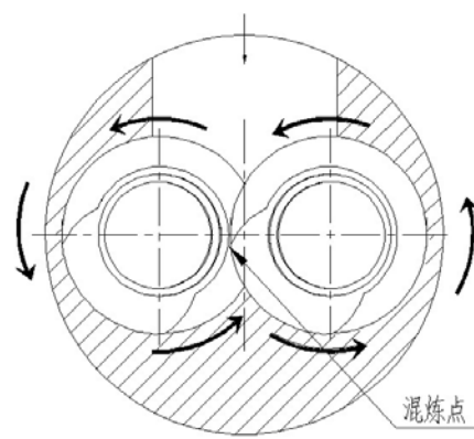
图2 锥形异向双螺杆工作原理
