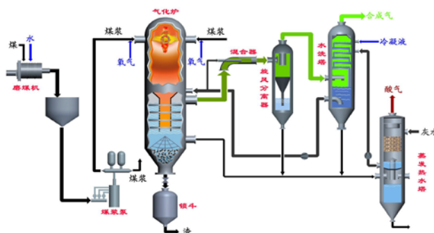
图 1 多喷嘴对置式水煤浆气化工艺流程图
