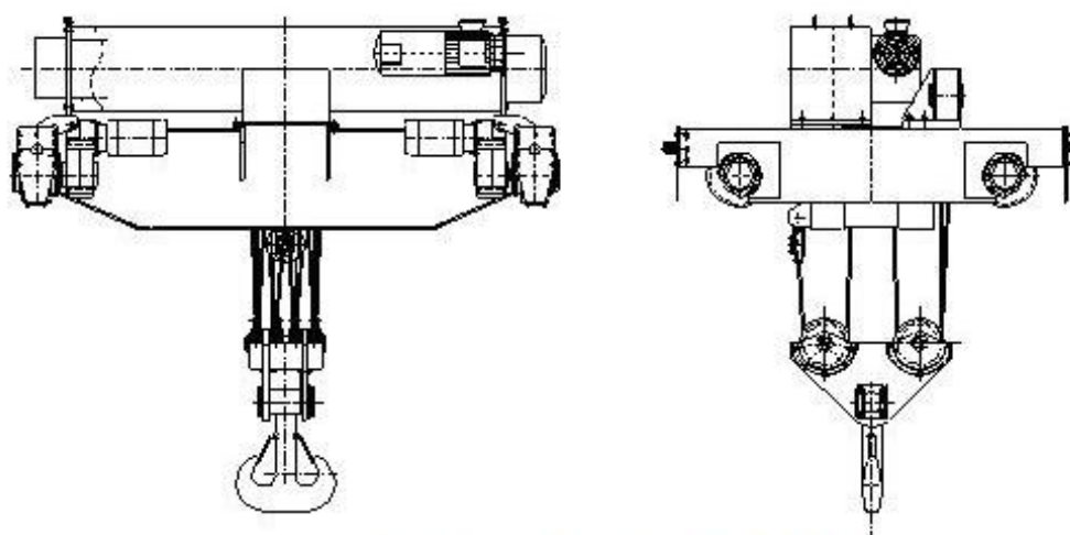
轻量化桥式起重机小车简图
