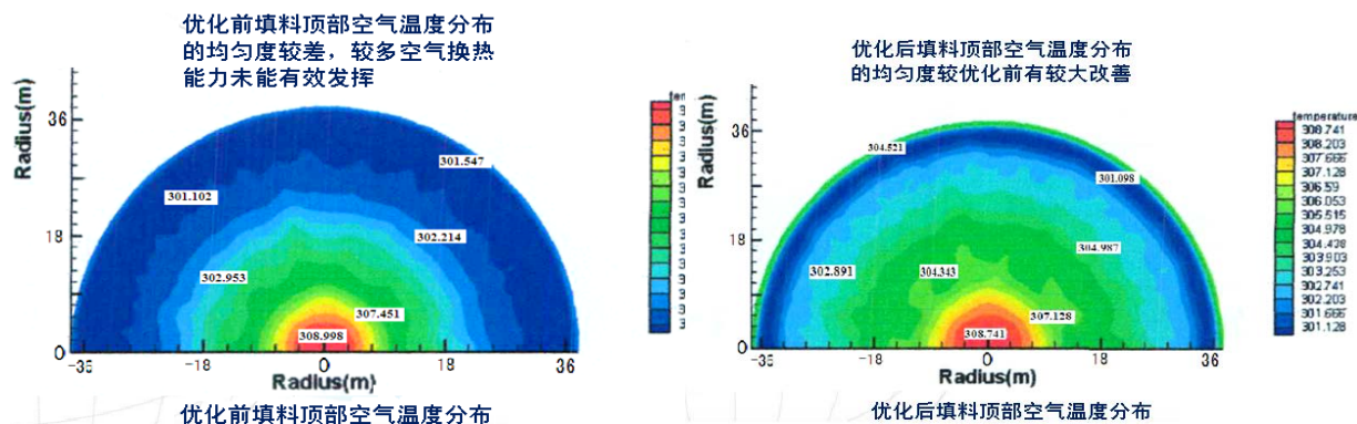
图1 自然通风逆流湿式冷却塔风水匹配强化换热技术实施效果对比图
