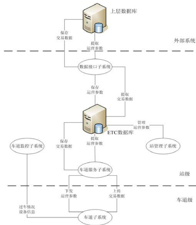
图 2 电子不停车收费系统原理简图
