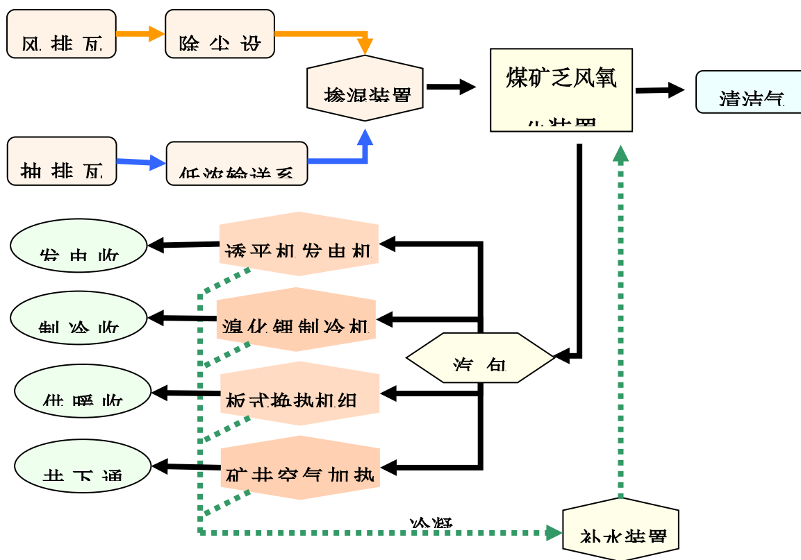
图 3 乏风氧化装置工艺流程图
