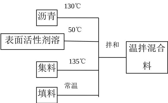
图 1 温拌沥青混合料工艺流程
