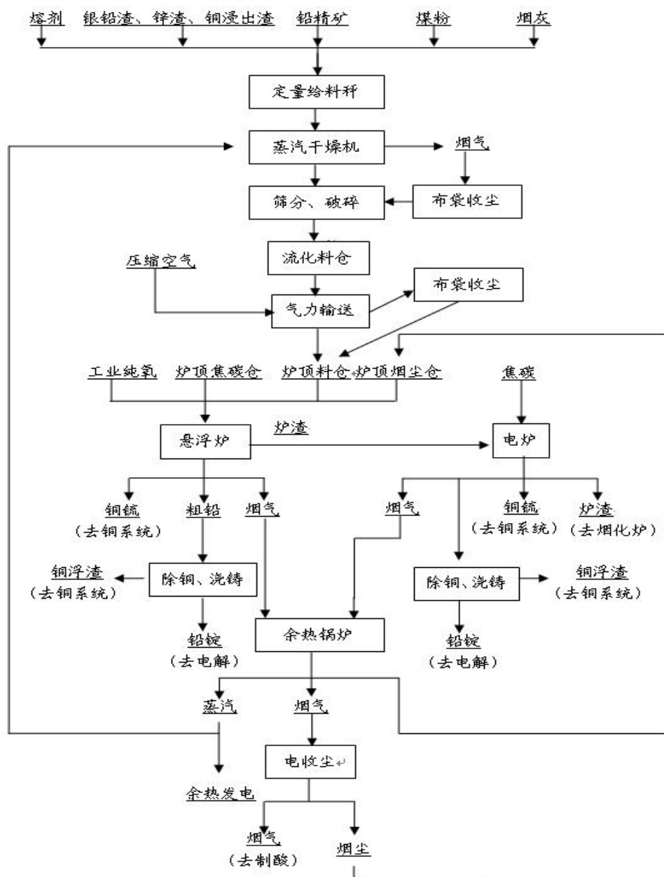
图 1 铅闪速熔炼工艺流程图
