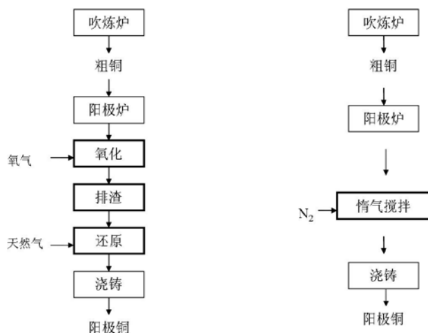
图 1 传统火法精炼工艺流程图图 2 新火法精炼工艺流程图
