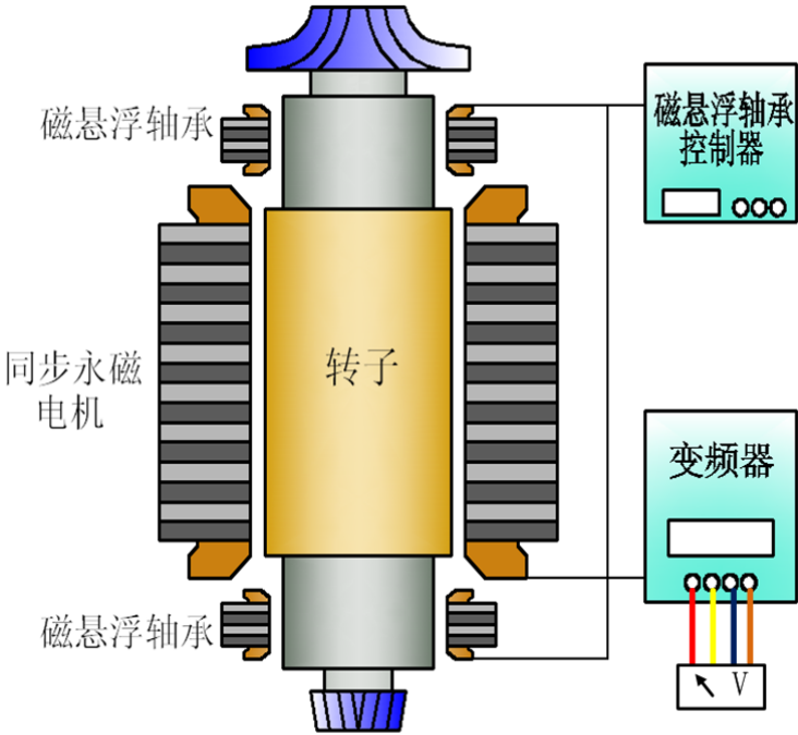
图 1 磁悬浮离心式鼓风机原理简图
