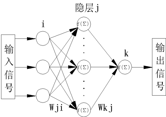
图2-3 前向型神经网络拓扑结构
