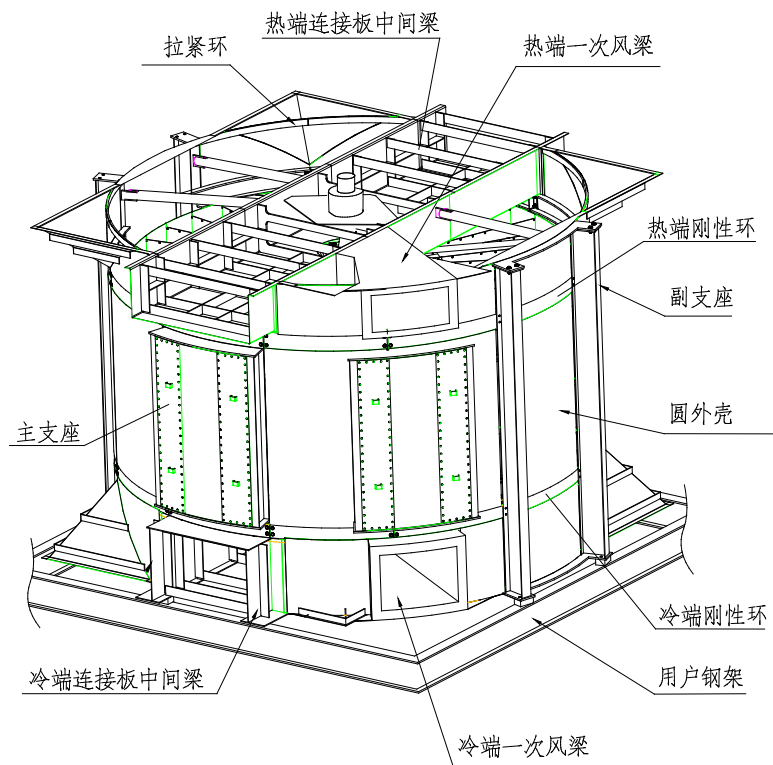
图 2 图 2 空气预热器立体图
