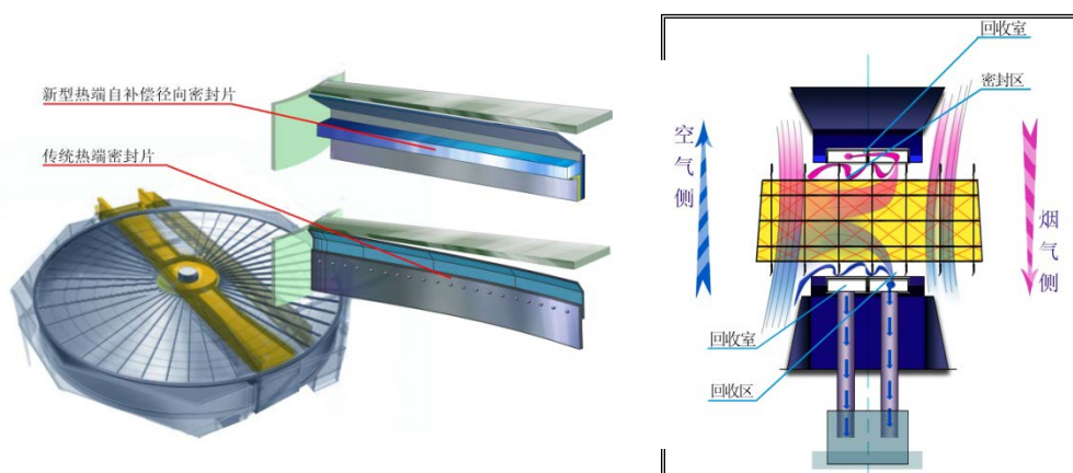
图2内部径向补偿间隙密封片示意图3漏风回收系统简图
