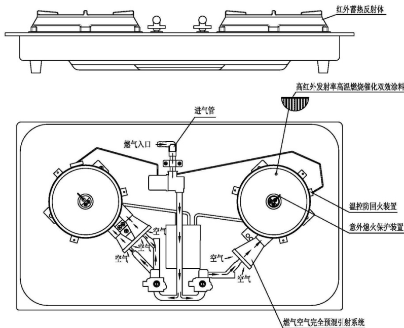
图 1 红外多孔陶瓷节能灶原理示意图
