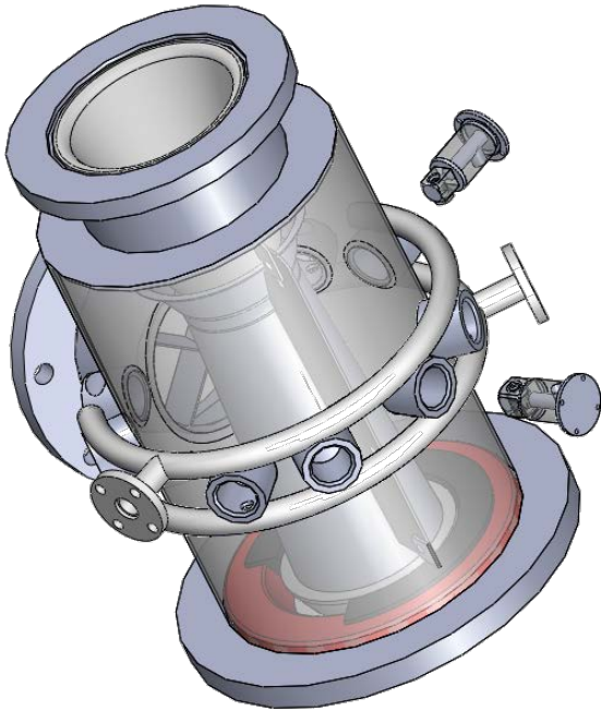
图 3：染液喷洒装置
