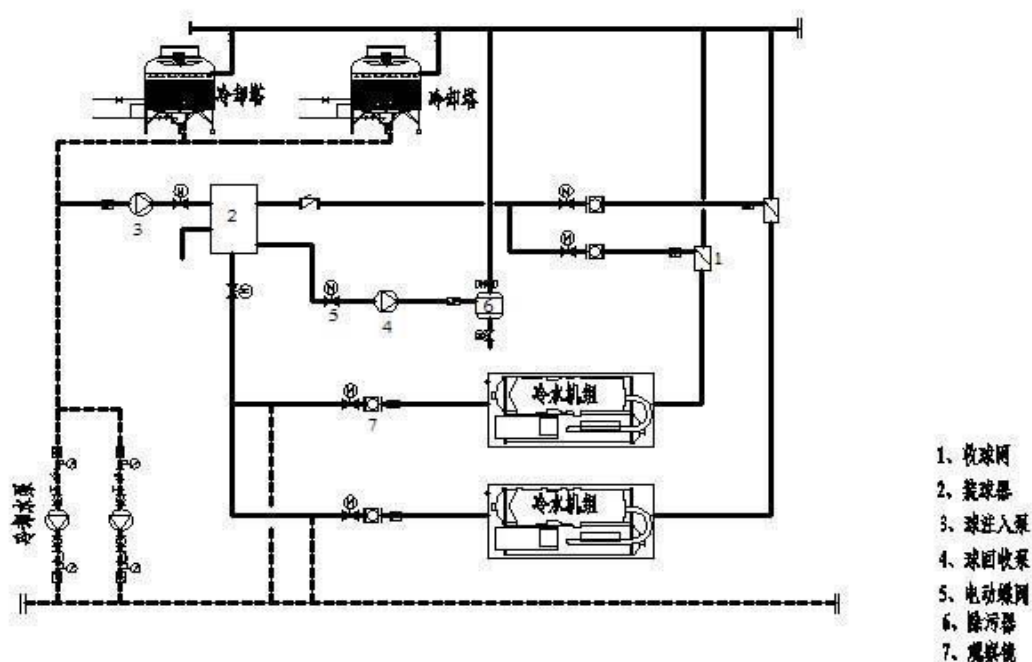
JSH-CTCS-II 系统原理图
