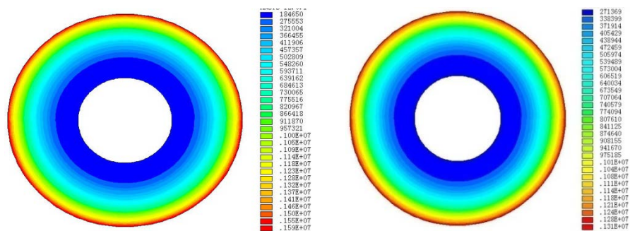
铜管的电流密度
