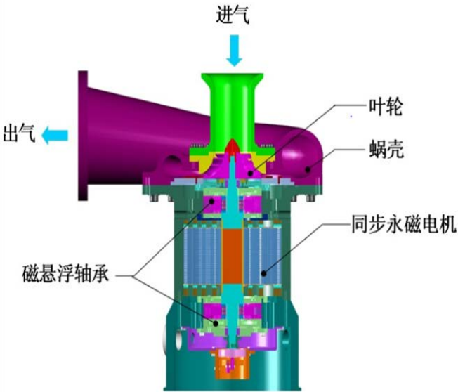
图 2 磁悬浮离心式鼓风机主机结构示意图
