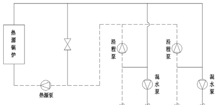
图3 工艺流程图
