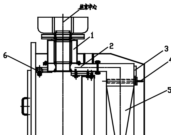
图 1 环吹风结构
