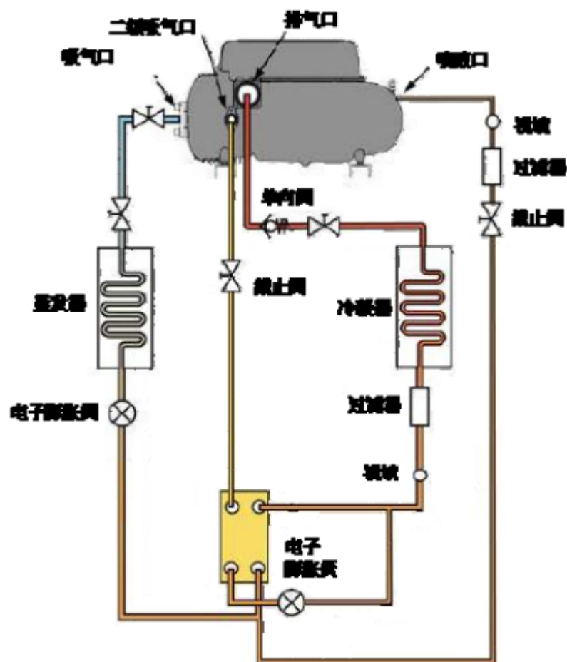
带过冷器设计的系统原理图
