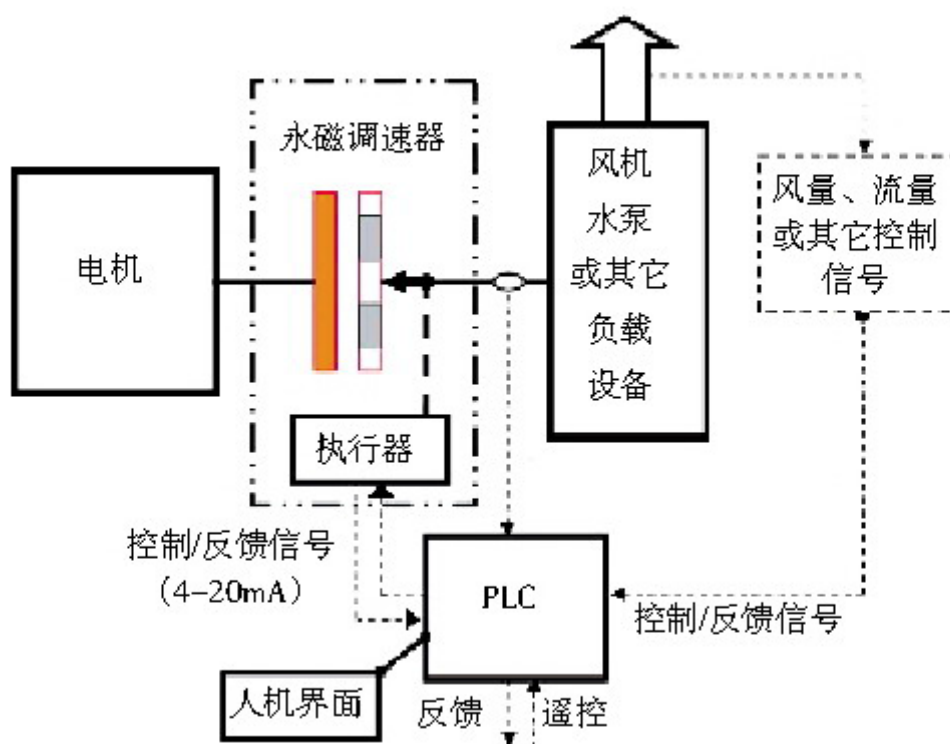
ASD 自动化控制流程图
