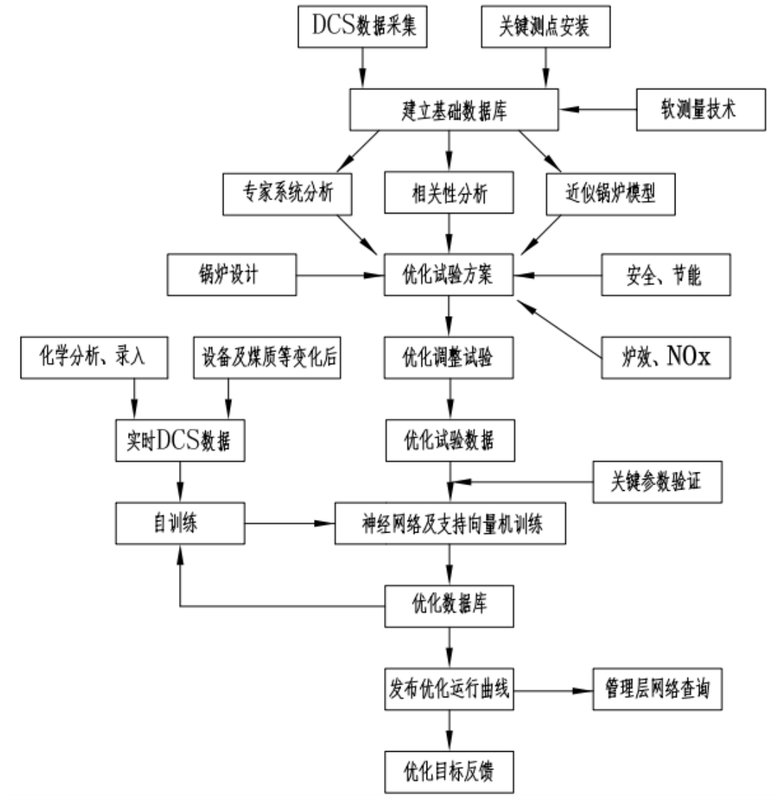
图 1 锅炉节能监测及系统优化流程图
