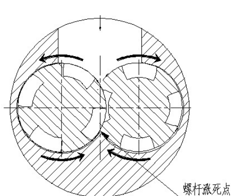
图1 锥形异向双螺杆工作原理简图
