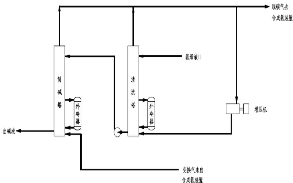
图2 环保型变换气制碱外冷碳化塔清洗新工艺流程示意图（无角阀流程）
