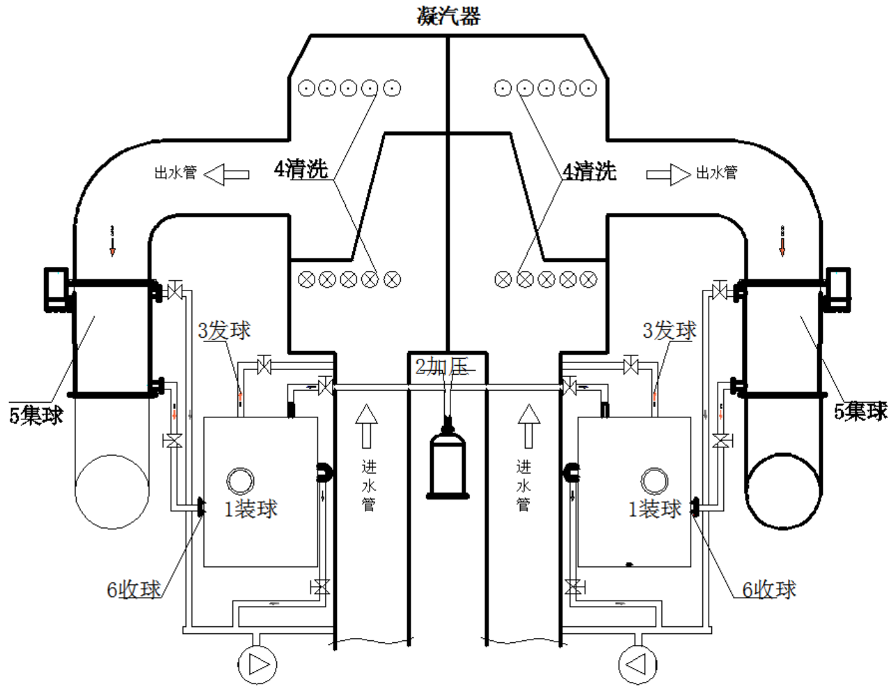
图2凝汽器真空保持节能系统主要设备简图
