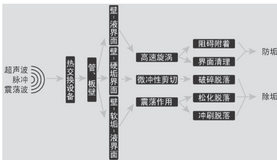
图 2 高速微涡效应防垢除垢作用图
