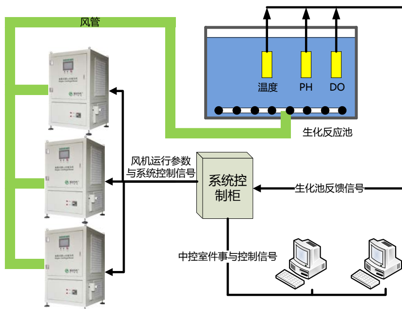
图 4 磁悬浮离心式鼓风机系统应用示意图
