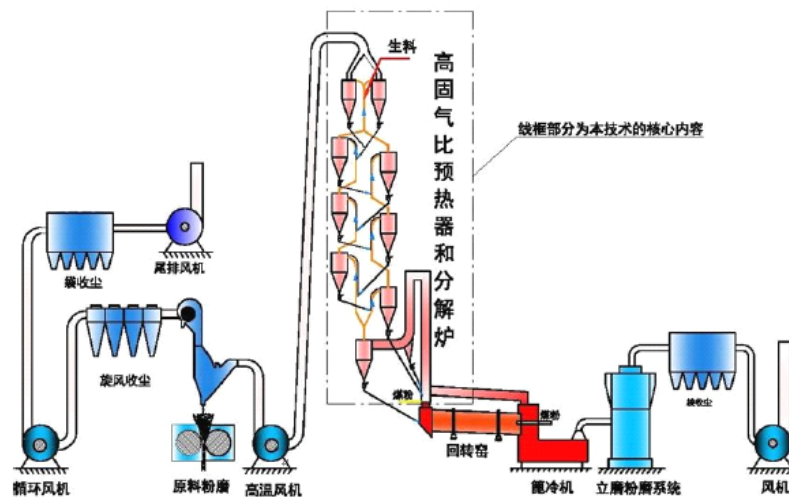
图 1 高固气比水泥煅烧技术工艺流程图
