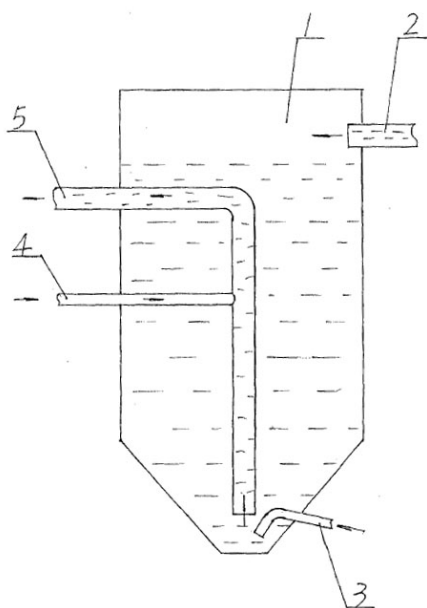
图 1 酸钠溶液微扰动平推流晶种分解技术流程图
