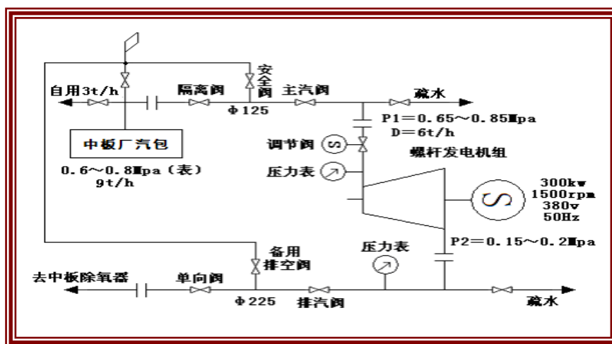
图 2 应用螺杆膨胀机的系统工艺流程图
