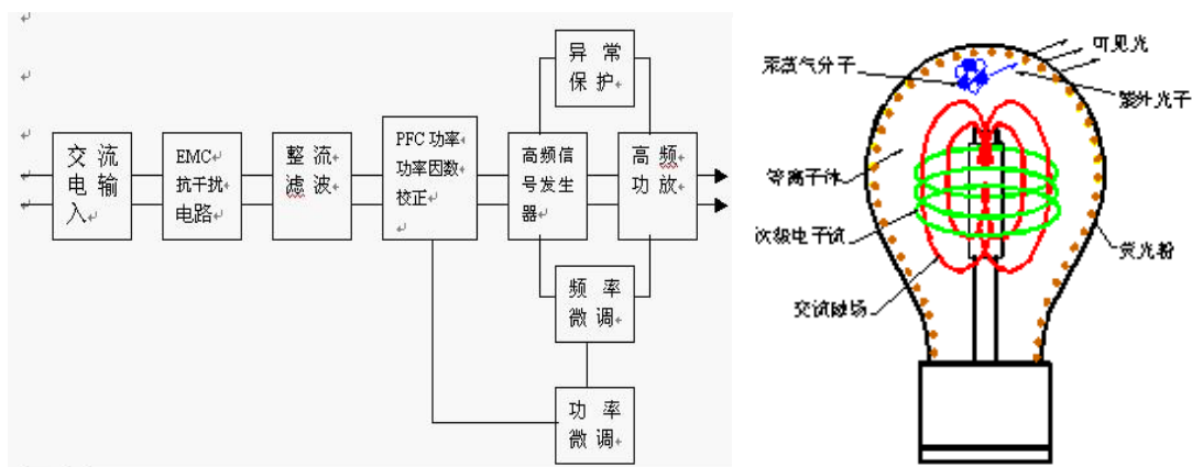
图1 内耦合无极灯工作原理图
