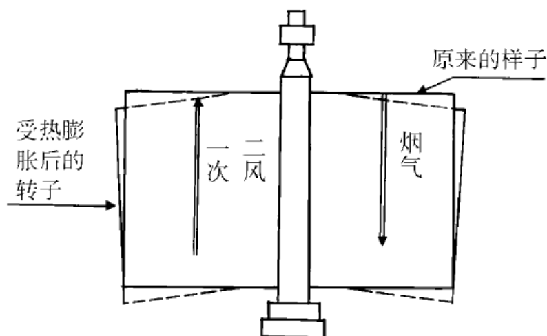
图 1 空预器转子受热前后膨胀对比图
