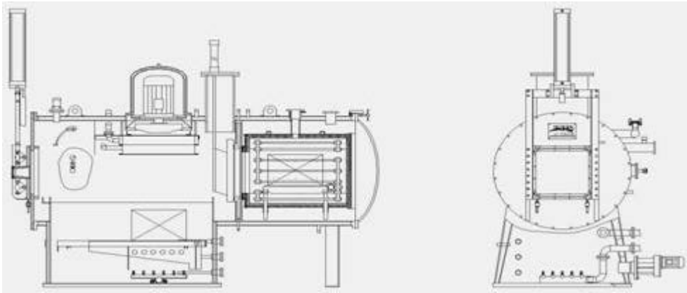
图 1 智能真空渗碳淬火炉设备简图
