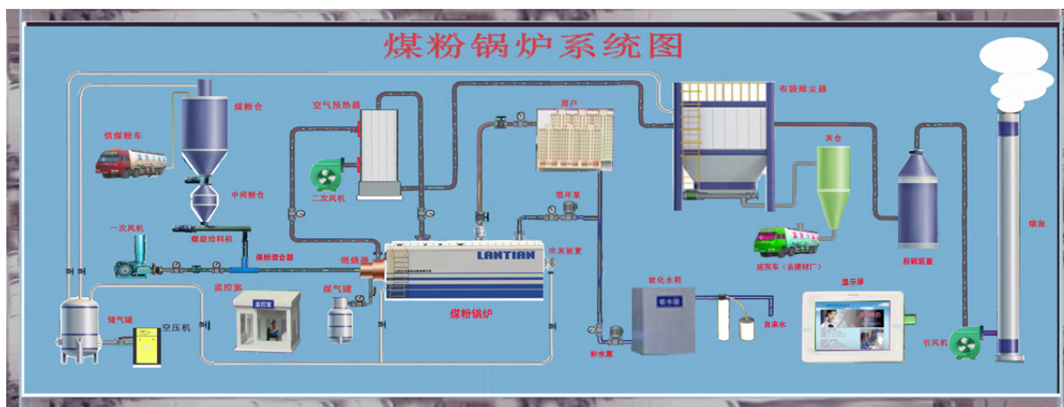
图1 新型高效煤粉工业锅炉系统技术流程图
