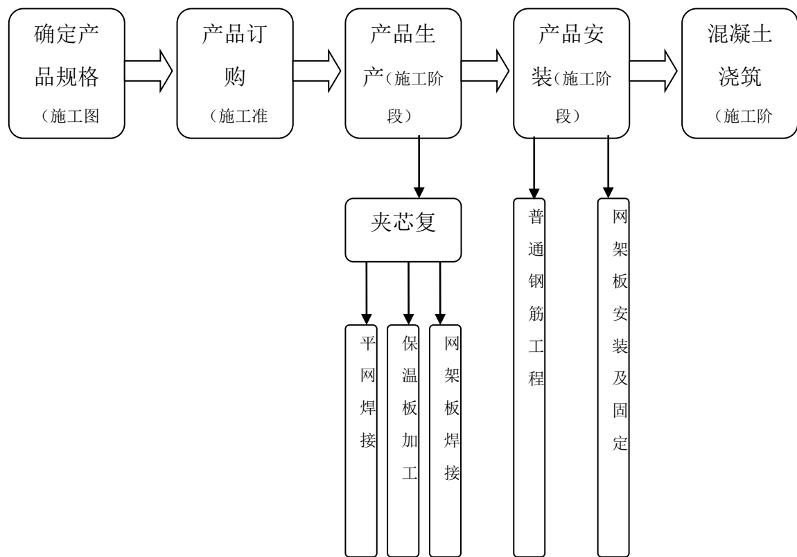
图2 夹芯复合轻型结构体系工艺流程
