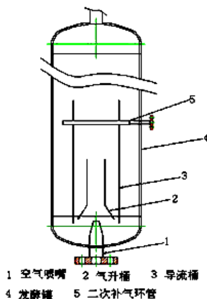
图 2 气升式二次补气发酵原理图
