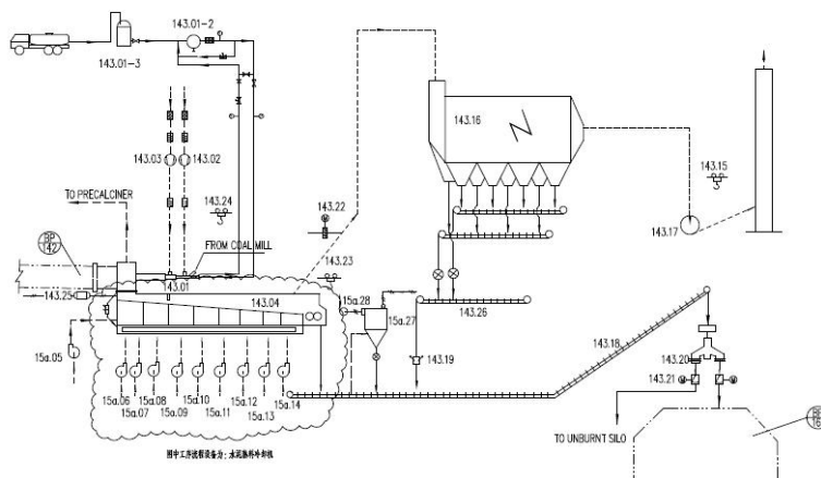
图 1 水泥窑熟料冷却机工艺流程图
