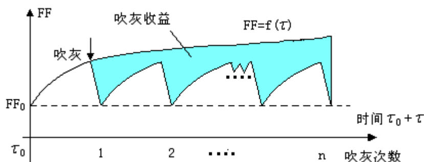
图 2-4 吹灰收益与吹灰频率的关系示意图
