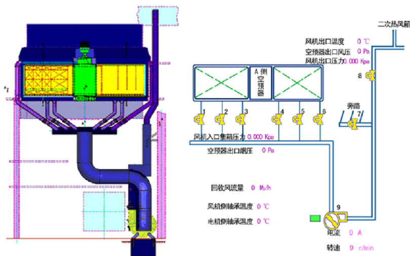
图 1 回转式空气预热器密封节能技术工艺流程
