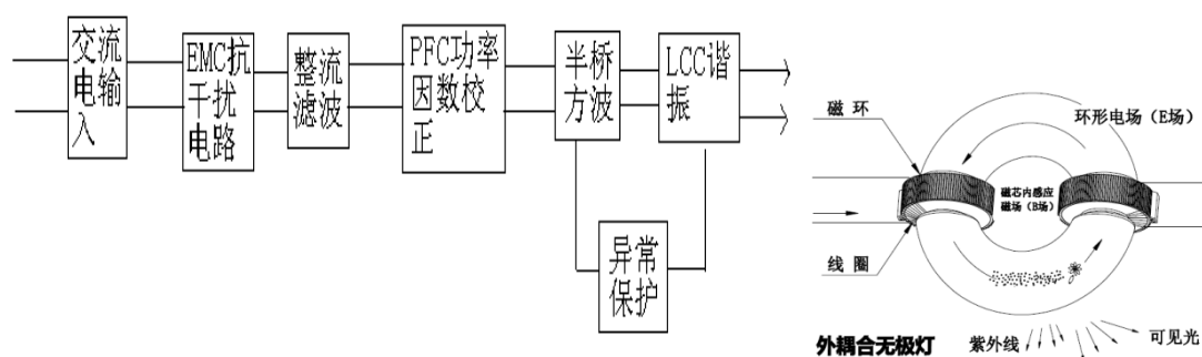
图 2 外耦合无极灯工作原理图
