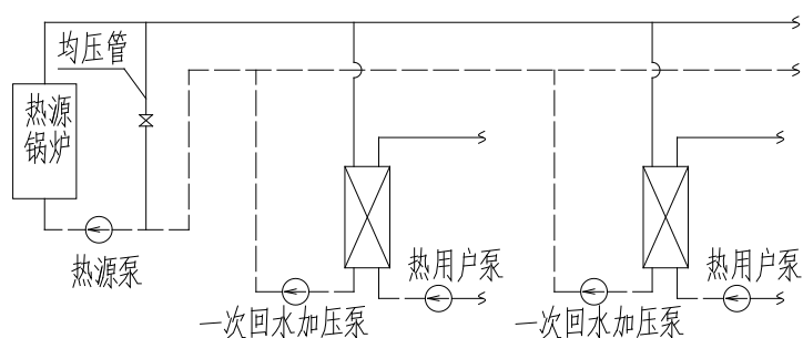
图2 工艺流程图
