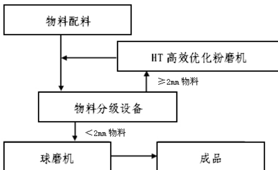
图2 高效优化粉磨节能技术工艺流程简图
