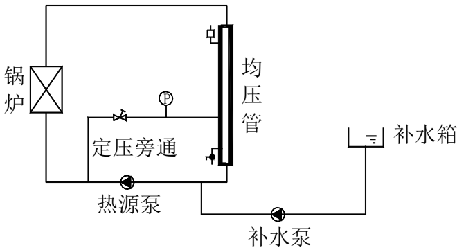
图1 补水定压示意图
