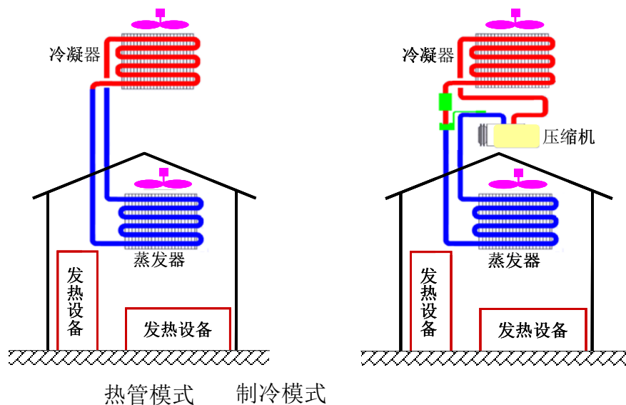
图 1 技术原理图
