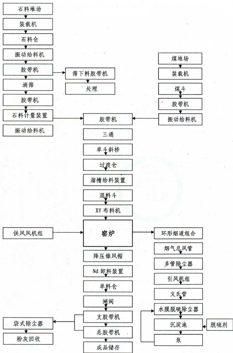
图 1-1 工艺流程图
