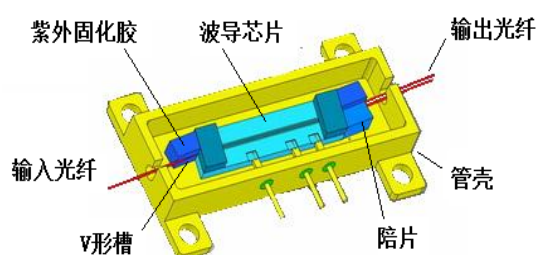
图 3 专用光电子器件结构
