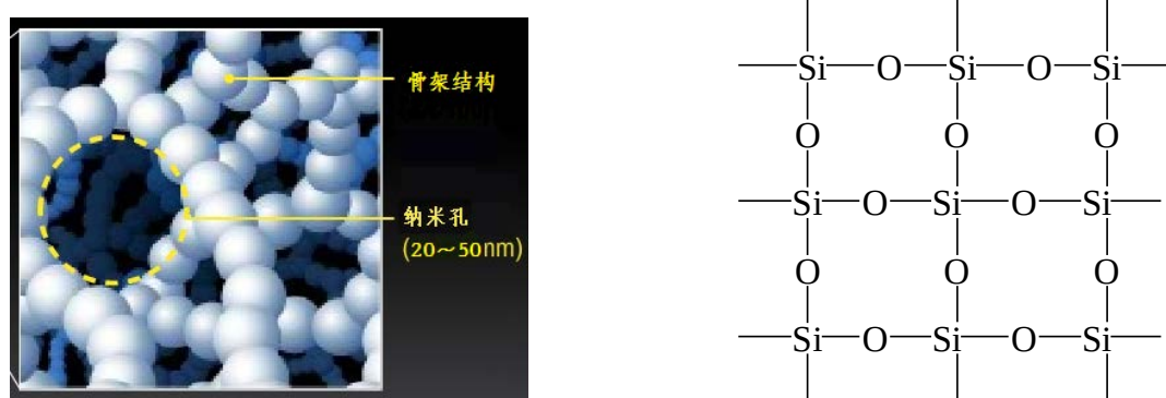
图 1 气凝胶超级绝热保温材料的立体结构图和分子结构图
