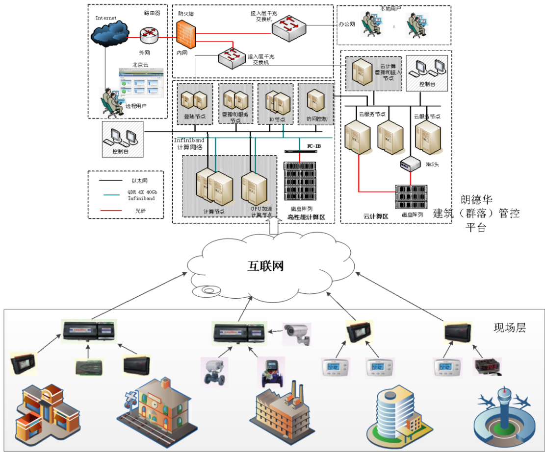
图 建筑（群落）能源动态管控优化系统技术硬件架构图
